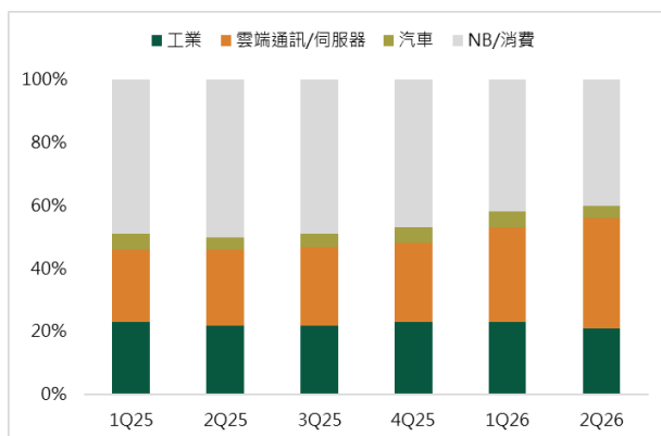
圖：產品組合
